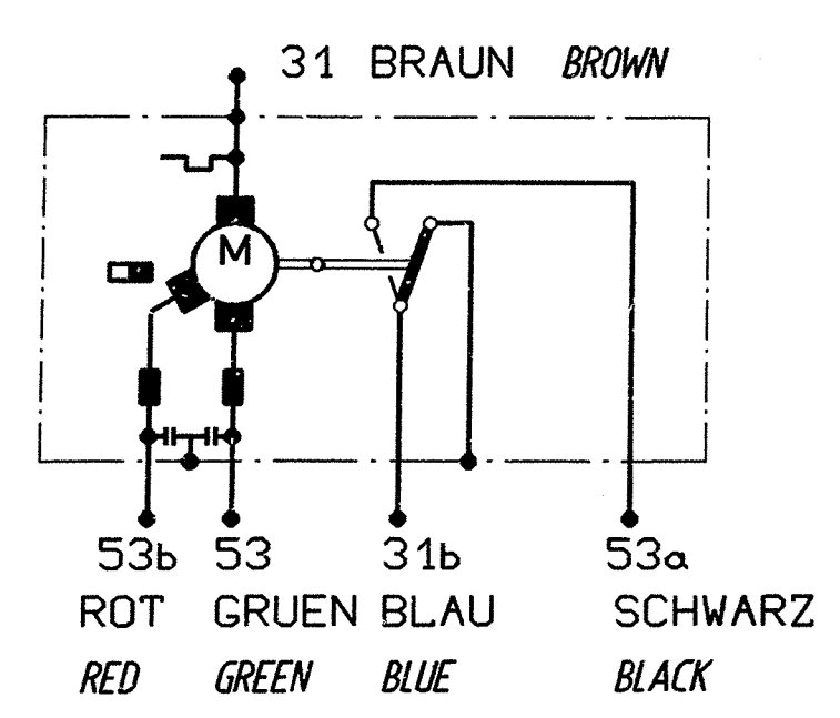
SCHALTBILD CIRCUIT DIAGRAM
